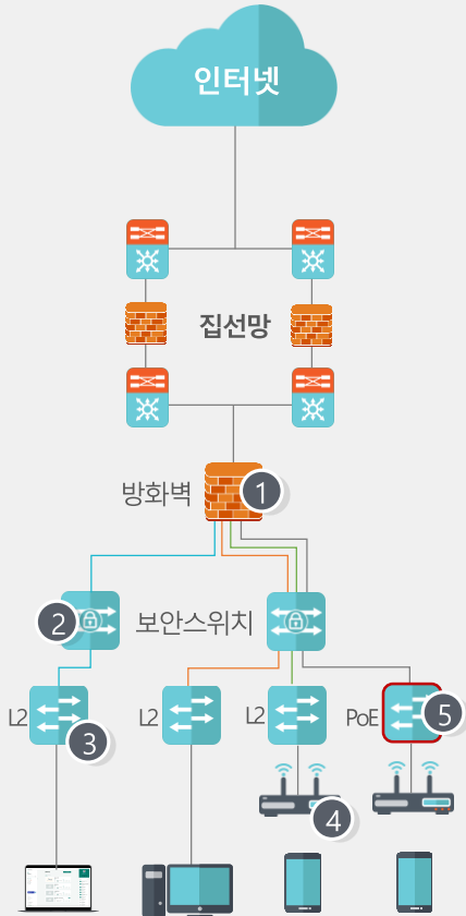
스쿨넷 구성도
